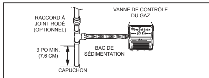
FIGURE 12. CONDUITES DE GAZ AVEC CONNECTEUR FLEXIBLE.
